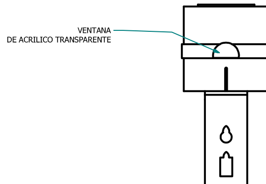
VISTA LATERAL ESC: 1 : 4
