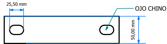
DETALLE ABRAZADERA ESC: ( 1 : 4 )
