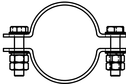
VISTA FRONTAL ESC: ( 1 : 4 )
