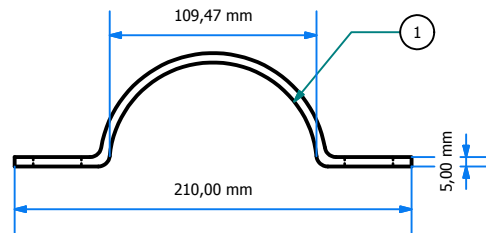
DETALLE ABRAZADERA ESC: ( 1 : 4 )
