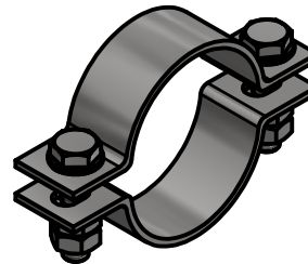
VISTA ISOMETRICA ESC: ( 1 : 5 )
