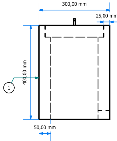
VISTA DE PERFIL ESC: 1 :10
