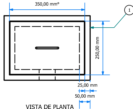
VISTA DE PLANTA ESC:1 :10
