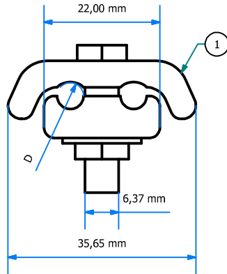
VISTA FRONTAL ESC: 1 : 1
