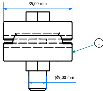
VISTA FRONTAL ESC: 1 : 1
