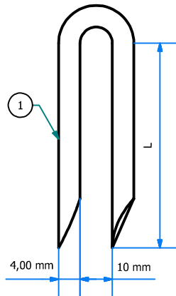
VISTA FRONTAL ESC: 1 : 1
