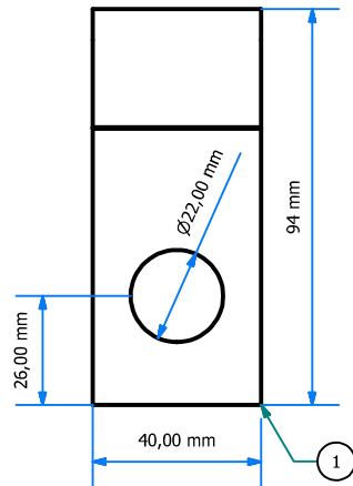
VISTA FRONTAL ESC: 1 : 2
