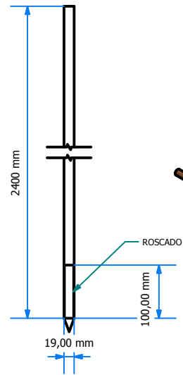
VISTA FRONTAL ESC: 1 : 10
