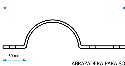
ABRAZADERA PARA SOPORTE VISTA FRONTAL ESC: 1 : 4
