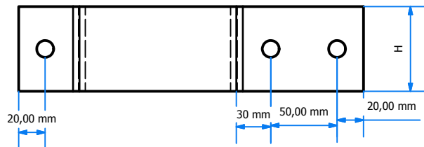
VISTA DE PLANTA ESC: 1 : 4
