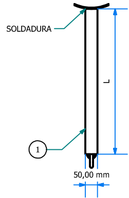
VISTA FRONTAL ESC: 1 : 16
