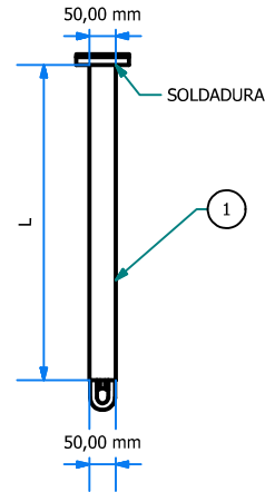
VISTA DE PERFIL ESC: 1 : 16
