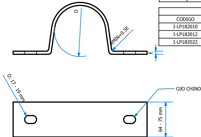
VISTA DE PLANTA ESC: 1 : 5
