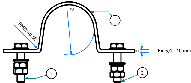
VISTA FRONTAL ESC: 1 : 5
