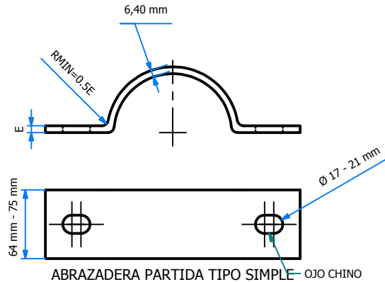
ABRAZADERA PARTIDA TIPO SIMPLE ESC: 1 : 5
