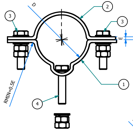
VISTA FRONTAL ESC: 1 : 5
