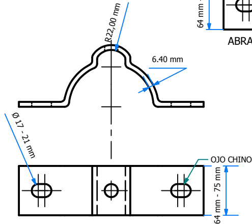
ABRAZADERA PARTIDA TIPO CAS ESC: 1 : 5
