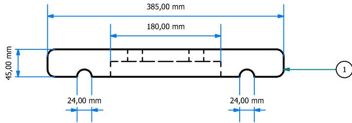
VISTA FRONTAL ESC: 1 : 6
