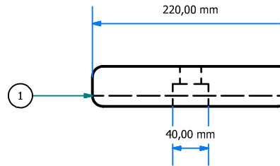
VISTA DE PERFIL ESC: 1 : 6
