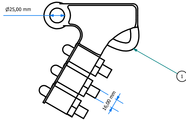
VISTA FRONTAL ESC: 1 : 4
