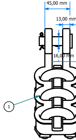
VISTA DE PERFIL ESC: 1 : 4
