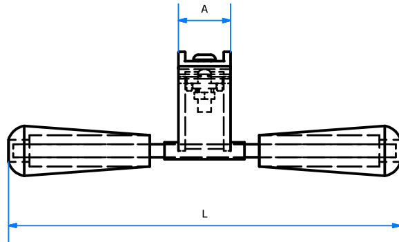
VISTA FRONTAL ESC: 1 : 4
