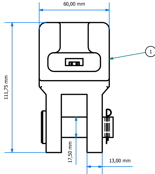
VISTA FRONTAL ESC: 1 :2
