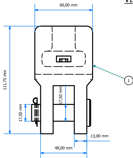
VISTA FRONTAL ESC: 1 : 2
