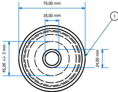
VISTA DE PLANTA ESC: 1 : 2.5
