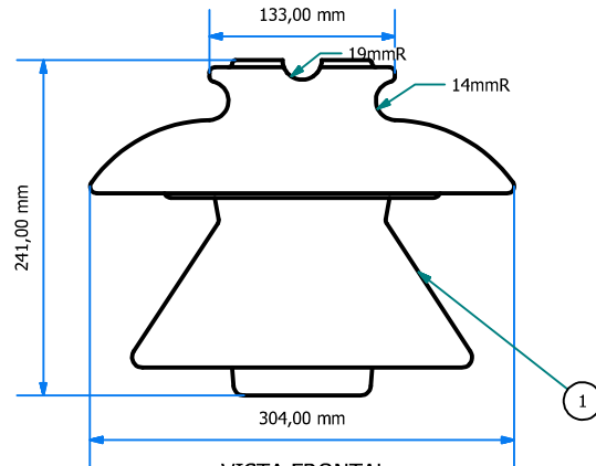
VISTA FRONTAL ESC : 1 : 6
