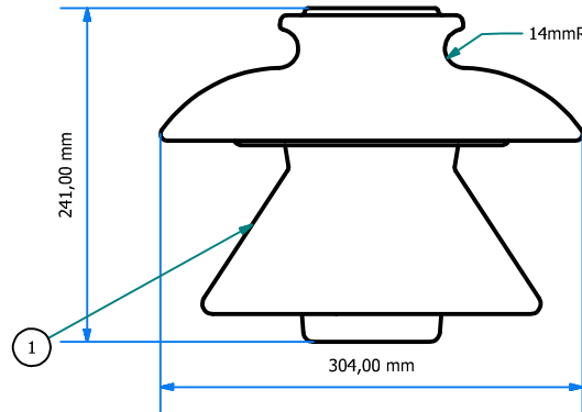
VISTA LATERAL ESC : 1 : 6
