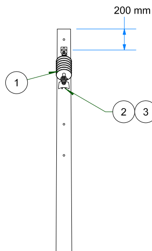
VISTA DE PERFIL ESC: 1 / 35
