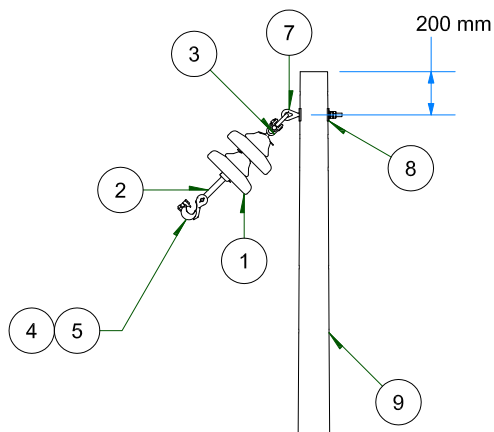
VISTA FRONTAL ESC: 1 / 35
