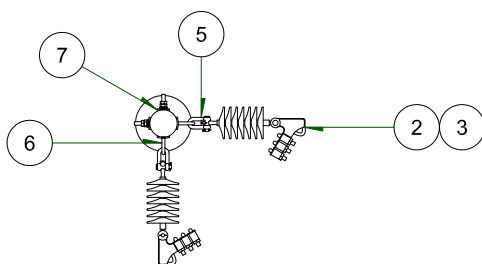
VISTA DE PLANTA ESC: 1 / 35
