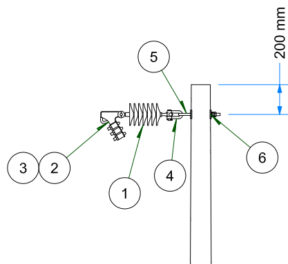
VISTA DE PERFIL ESC: 1 / 35
