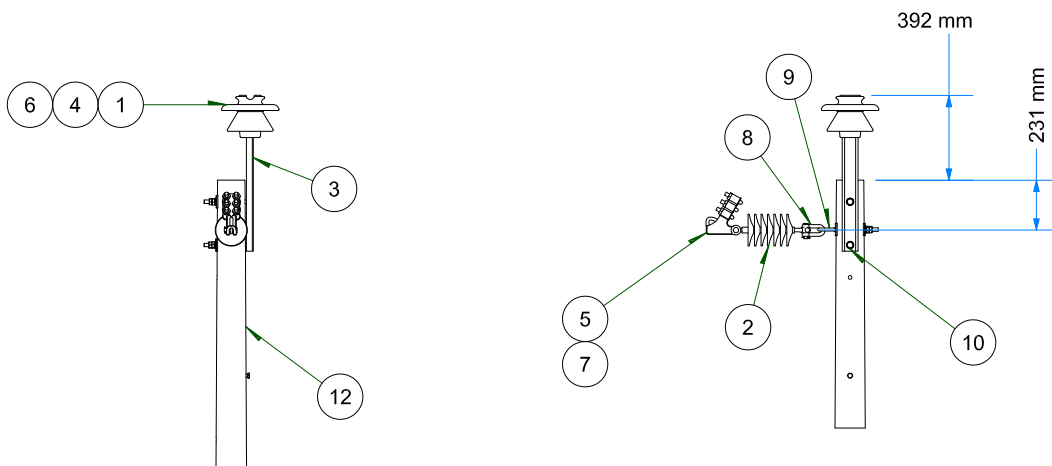
VISTA DE PERFIL ESC: 1 / 35
