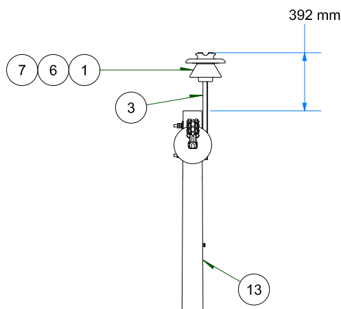
VISTA FRONTAL ESC: 1 / 35
