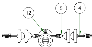
VISTA FRONTAL ESC: 1 / 35
