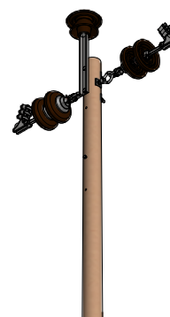
VISTA ISOMETRICA ESC: 1 / 50
