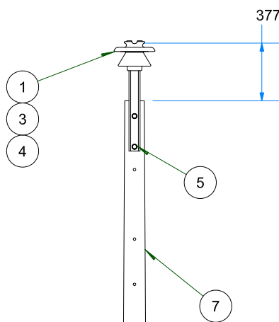
VISTA FRONTAL ESC: 1 / 35
