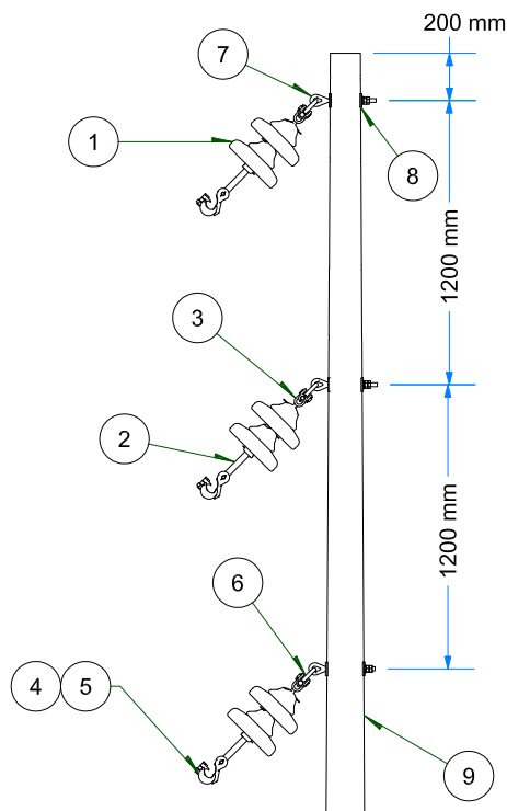
VISTA FRONTAL ESC: 1 / 35
