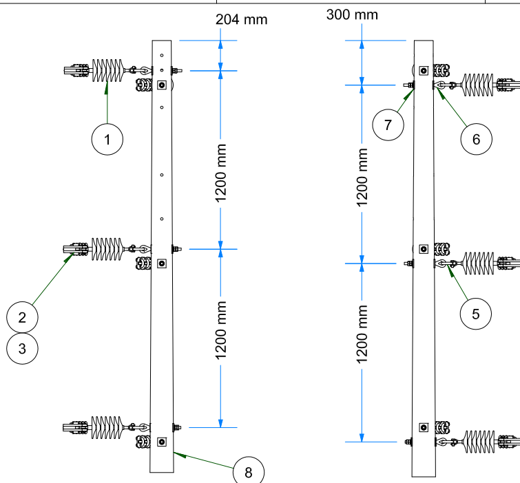
VISTA FRONTAL ESC: 1 / 35
