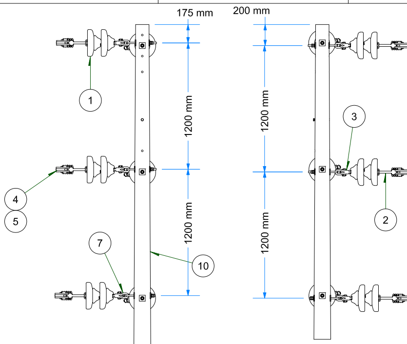
VISTA DE PERFIL ESC: 1 / 35
