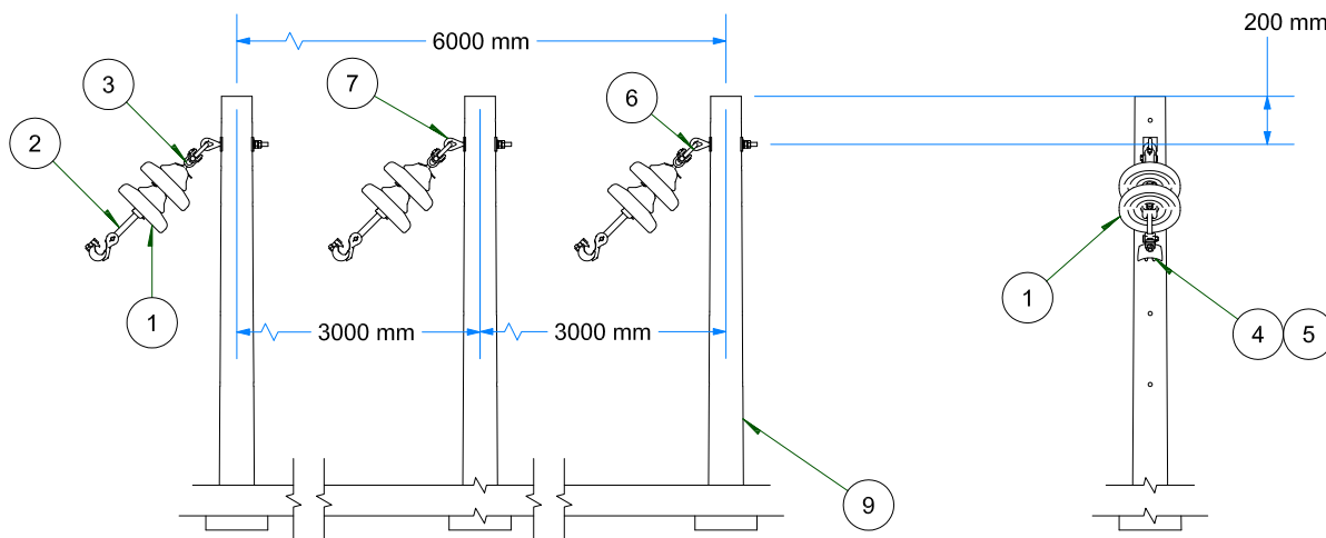
VISTA DE PERFIL ESC: 1 / 35
