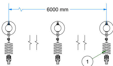
VISTA DE PLANTA ESC: 1 / 35
