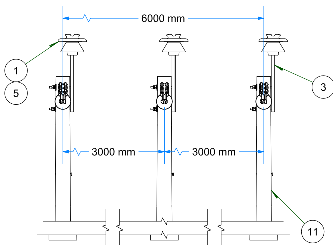
VISTA FRONTAL ESC: 1 / 35
