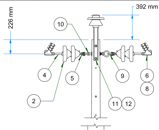
VISTA DE PERFIL ESC: 1 / 35
