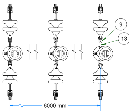
VISTA DE PLANTA ESC: 1 / 35
