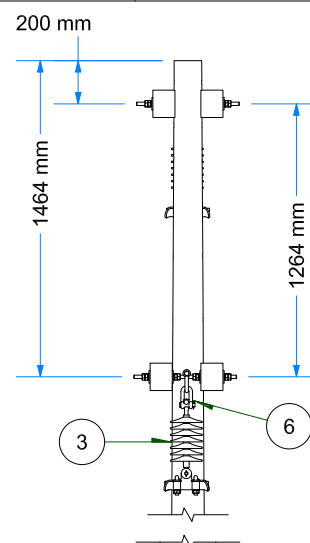
VISTA DE PERFIL ESC: 1 / 35
