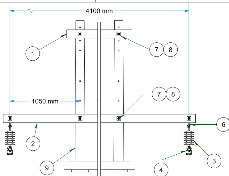
VISTA FRONTAL ESC: 1 / 35
