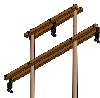
VISTA ISOMETRICA ESC: 1 / 75
