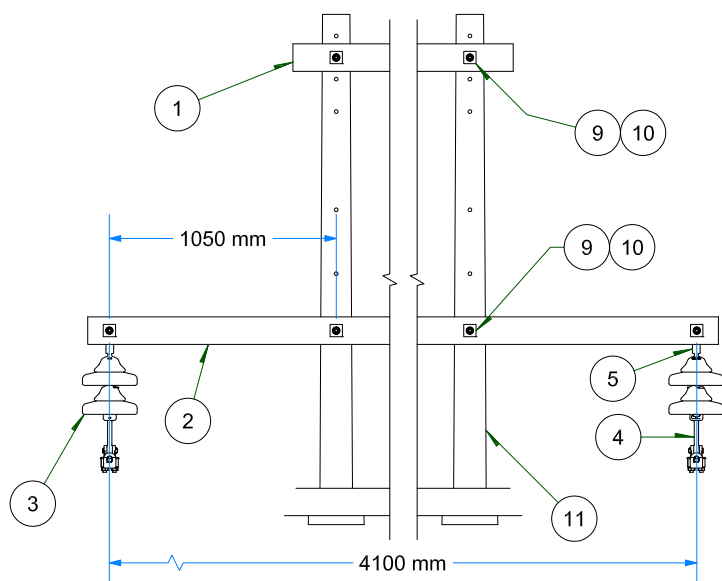
VISTA FRONTAL ESC: 1 / 35
