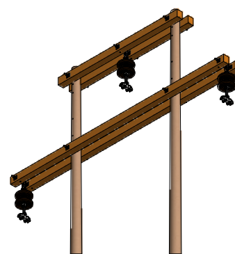
VISTA ISOMETRICA ESC: 1 / 75
