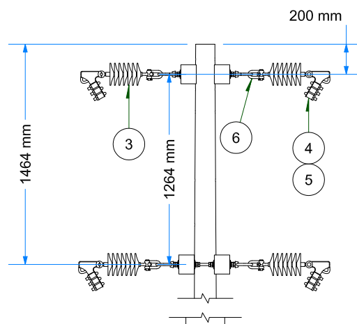
VISTA DE PERFIL ESC: 1 / 35
