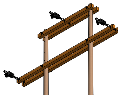
VISTA ISOMETRICA ESC: 1 / 75
