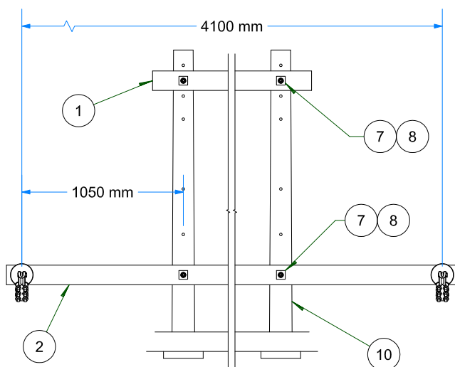
VISTA FRONTAL ESC: 1 / 35
