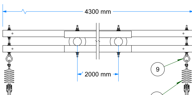
VISTA DE PLANTA ESC: 1 / 35
