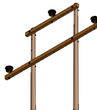
VISTA ISOMETRICA ESC: 1 / 75
