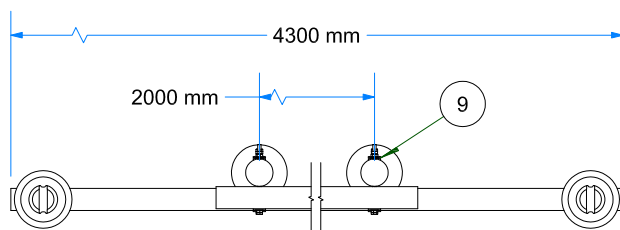
VISTA DE PLANTA ESC: 1 / 35
