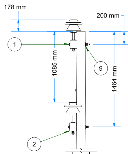
VISTA DE PERFIL ESC: 1 / 35
