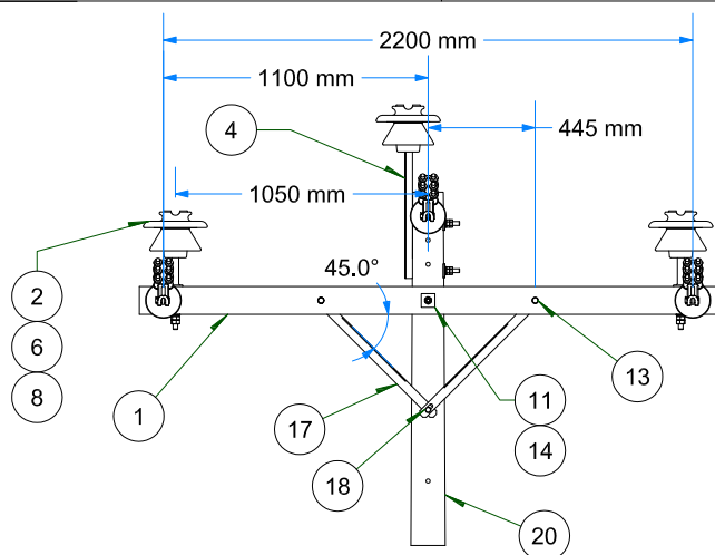
VISTA FRONTAL ESC: 1 / 35
