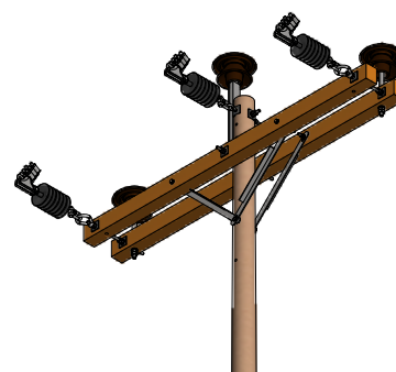
VISTA ISOMETRICA ESC: 1 / 50
