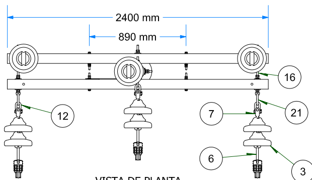
VISTA DE PLANTA ESC: 1 / 35
