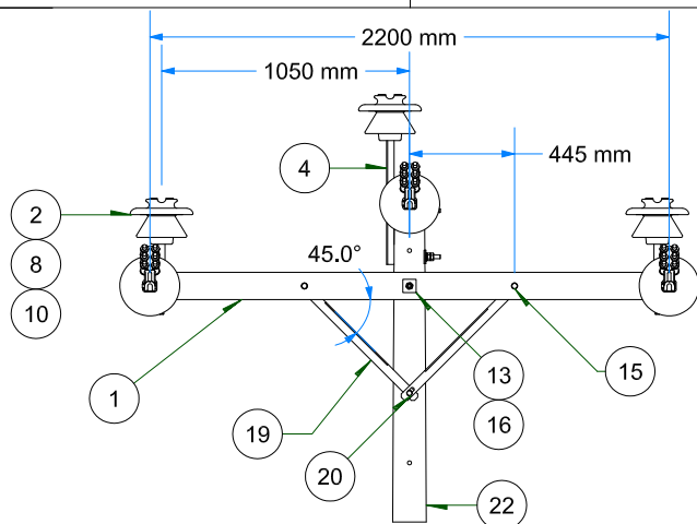
VISTA FRONTAL ESC: 1 / 35
