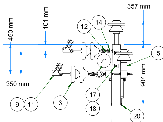
VISTA DE PERFIL ESC: 1 / 35
