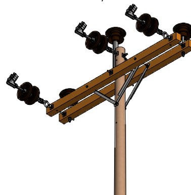
VISTA ISOMETRICA ESC: 1 / 50
