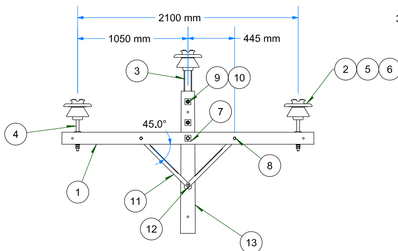
VISTA FRONTAL ESC: 1 / 35
