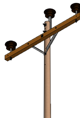
VISTA ISOMETRICA ESC: 1 / 50
