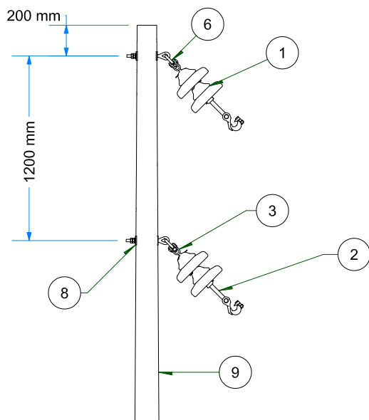
VISTA FRONTAL ESC: 1 / 35
