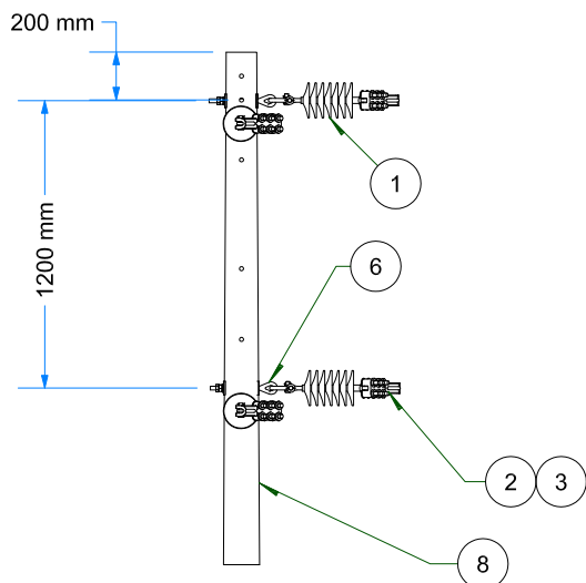
VISTA FRONTAL ESC: 1 / 35
