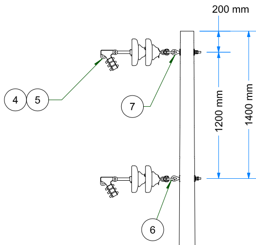
VISTA DE PERFIL ESC: 1 / 35
