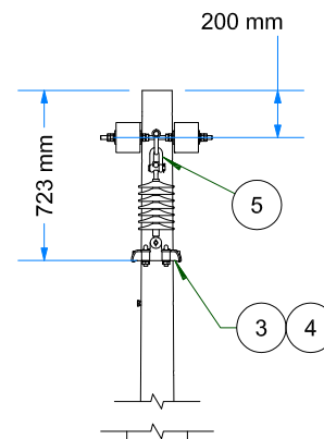
VISTA DE PERFIL ESC: 1 / 35
