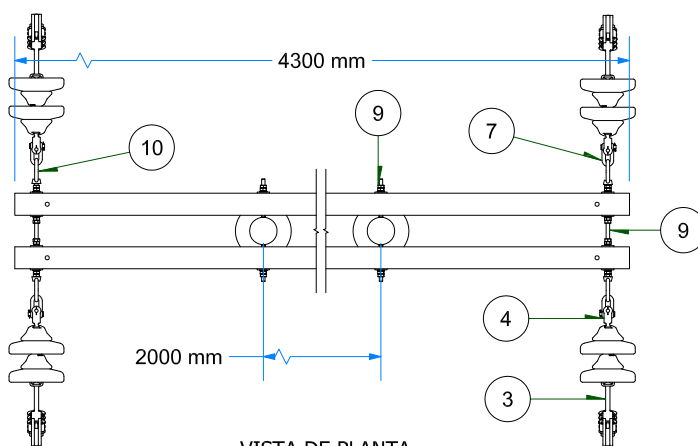
VISTA DE PLANTA ESC: 1 / 35
