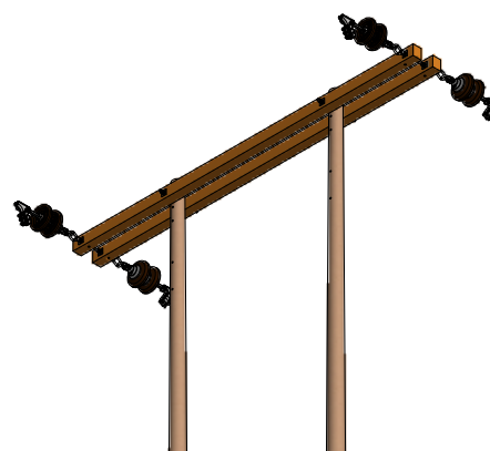
VISTA ISOMETRICA ESC: 1 / 75
