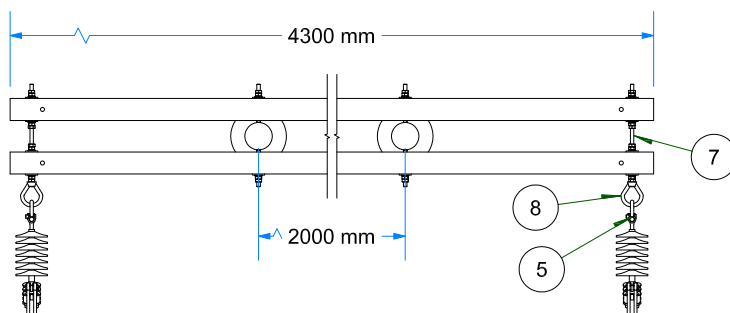
VISTA DE PLANTA ESC: 1 / 35
