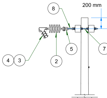
VISTA DE PERFIL ESC: 1 / 35
