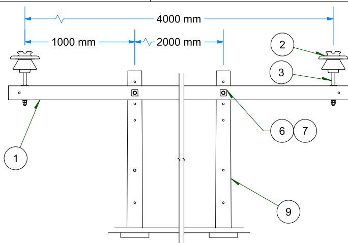
VISTA FRONTAL ESC: 1 / 35
