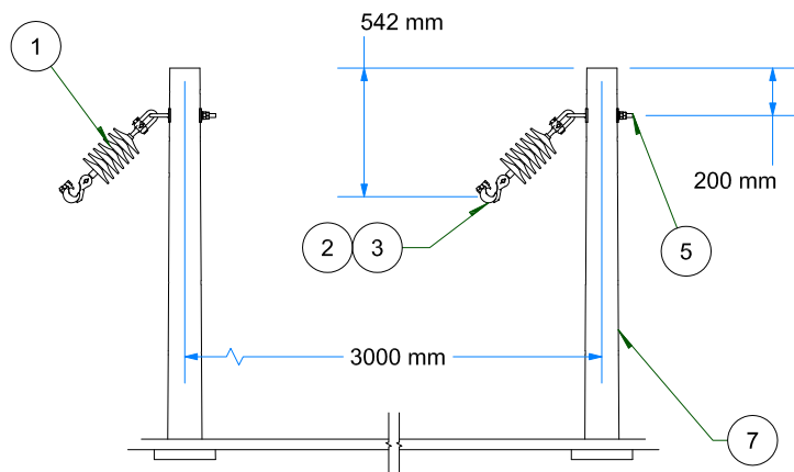
VISTA FRONTAL ESC: 1 / 35
