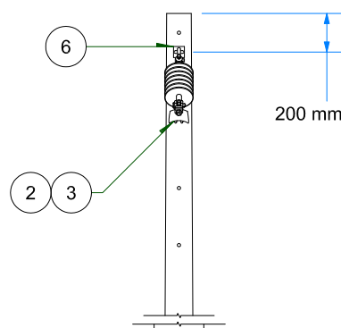
VISTA DE PERFIL ESC: 1 / 35
